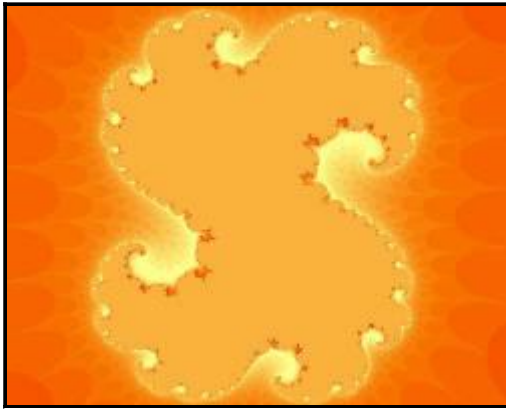
Juliova množina
