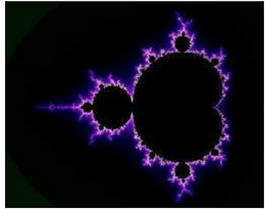
Mandelbrotova množina
