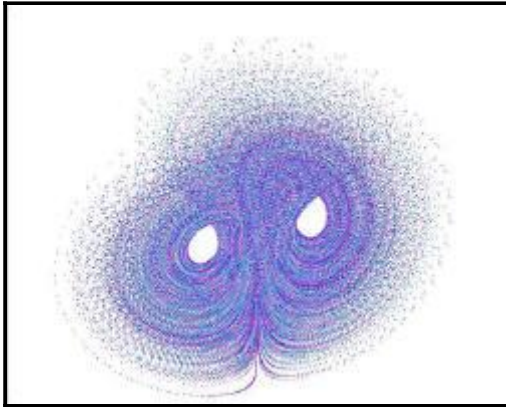
Lorenzův atraktor
