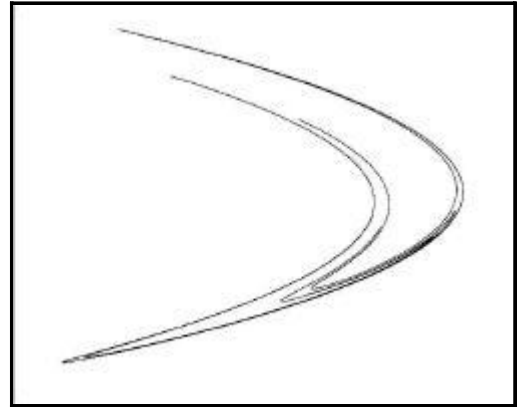
Hénonův atraktor
