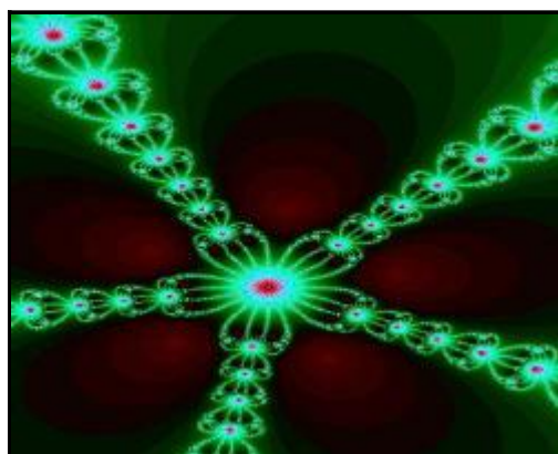
Newtonova množina
